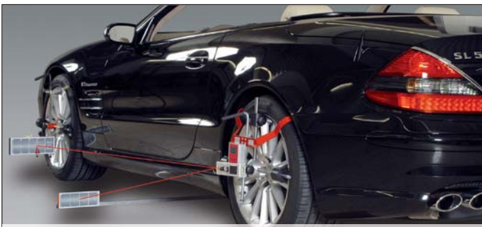
Hinterachsvermessung mit HD-10 EasyTouch
